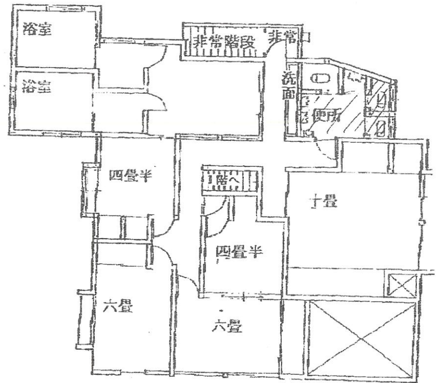
民宿ひとみ 2階平面図
